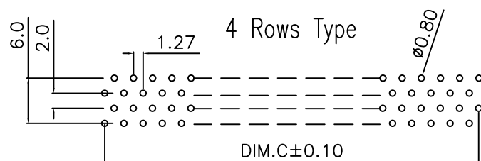
P. C. B. LAYOUT
