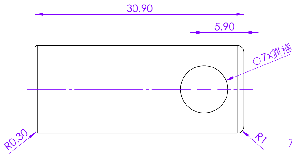
剖面圖 A-A 比例 3:1
