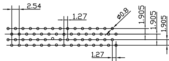
P.C.Board Layout
