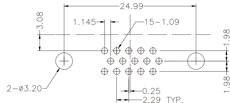
P.C.B. LAYOUT
