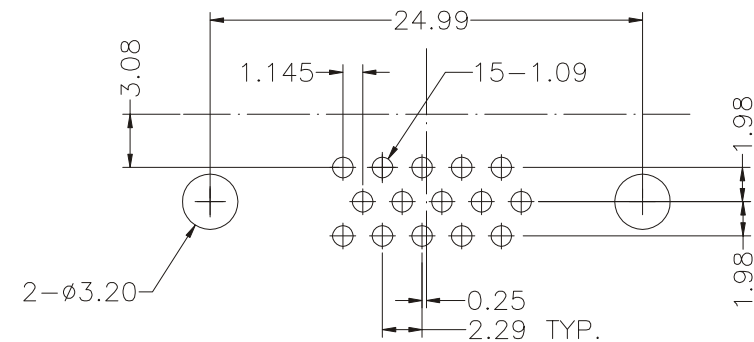
P.C.B. LAYOUT
