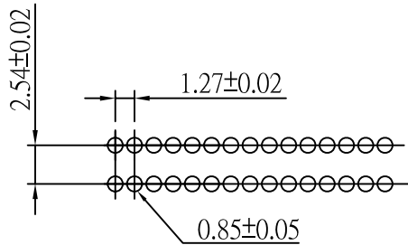
P.C.Board Layout
