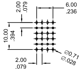
Press fit pin
