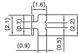
FITTING NAIL PLATE DIM.
