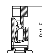
SECTION A-A SCALE 1:1
