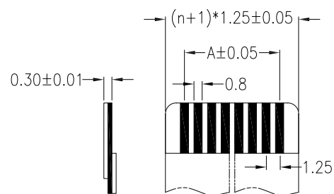
适用扁平电缆 (Proper cable)
