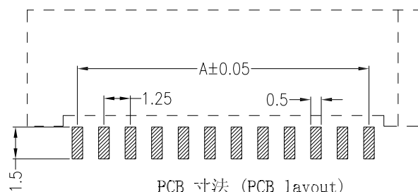
PCB 寸法 (PCB layout)
