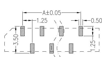
反针 PCB 寸法 Versa needle PCB layout R TYPE FOOT
