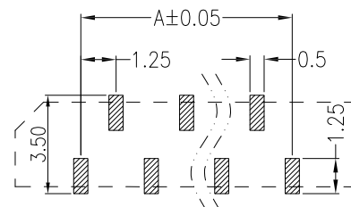
正针 PCB 寸法 Positive needle PCB layout L TYPE FOOT
