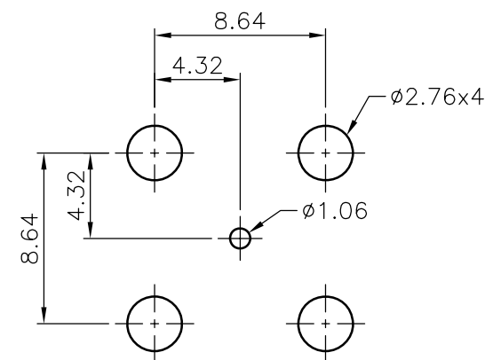
P.C.B. LAYOUT (印刷電路板配置)
