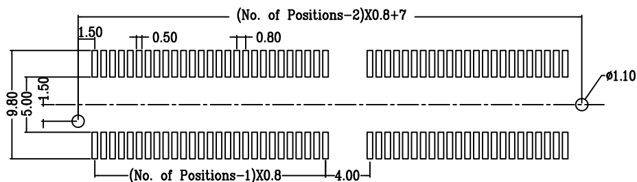
P.C.B.Layout
