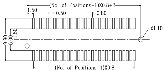
P.C.B.Layout
