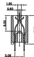
SEC A-A
