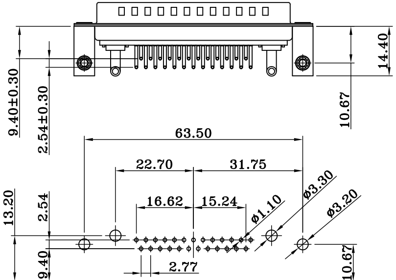
P.C.B LAYOUT
