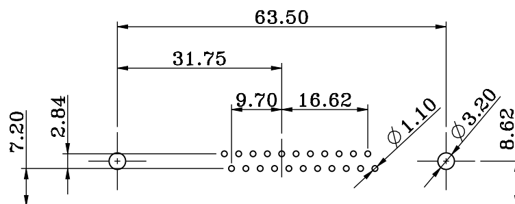
P.C.B. LAYOUT
