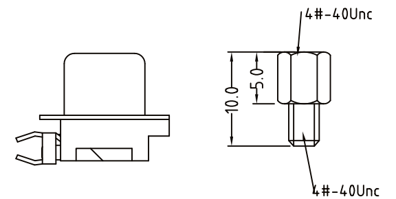
DW-SNHZ4-09
