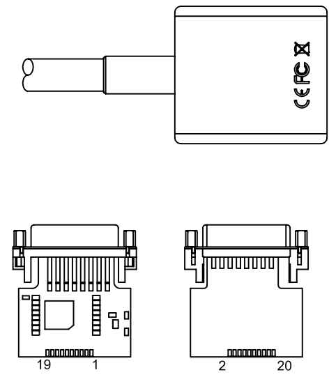
PCB'A
