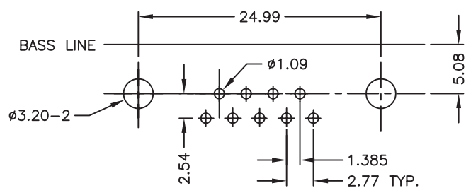
P.C.B. LAYOUT
