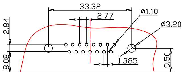
£ P.C.B EDGE RECOMMENDED P.C.B LAYOUT
