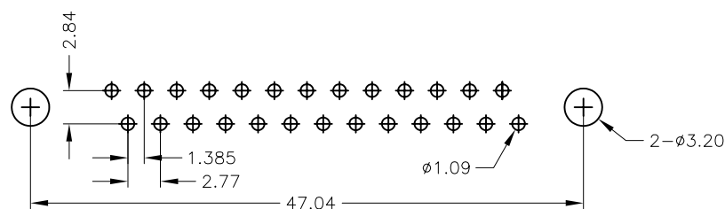
P.C.B. LAYOUT
