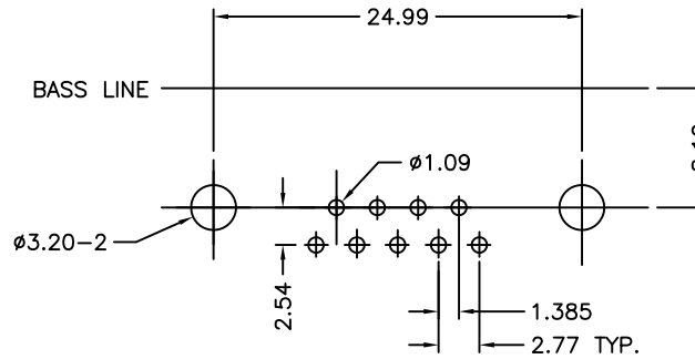
P.C.B. LAYOUT
