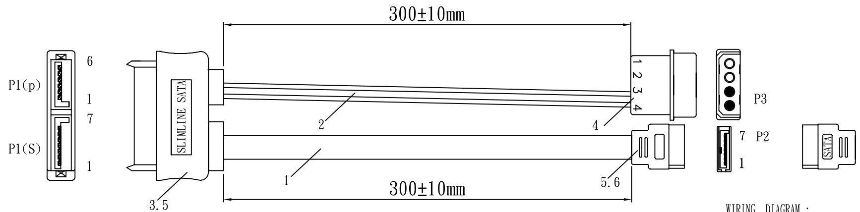
WIRING DIAGRAM :
