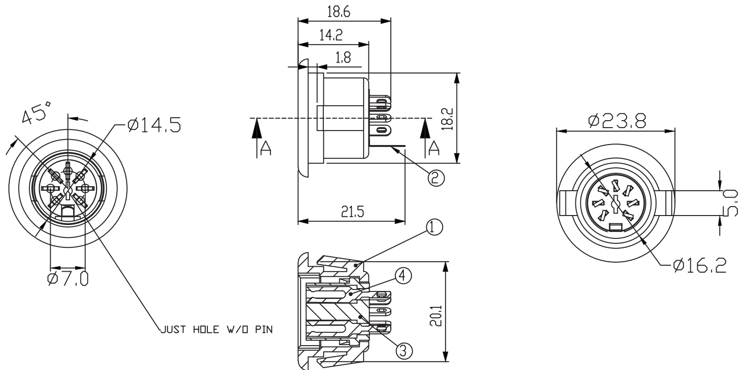
A-A SECTION
