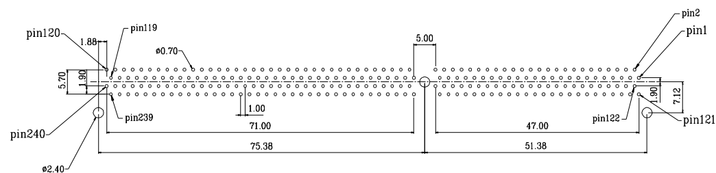
P.C.B. layout
