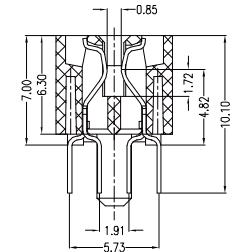
SECT A-A SCAL:3:1
