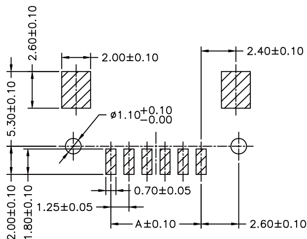
P.C.B. LAYOUT
