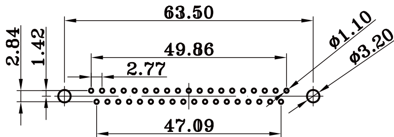
P.C.B LAYOUT
