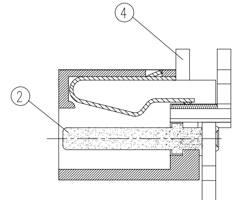
A-A SECTION
