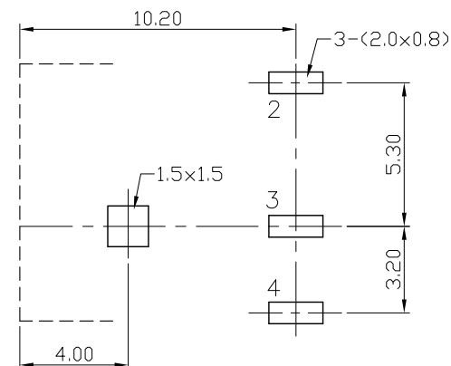
线路板开孔尺寸 P.C.B LAYOUT
