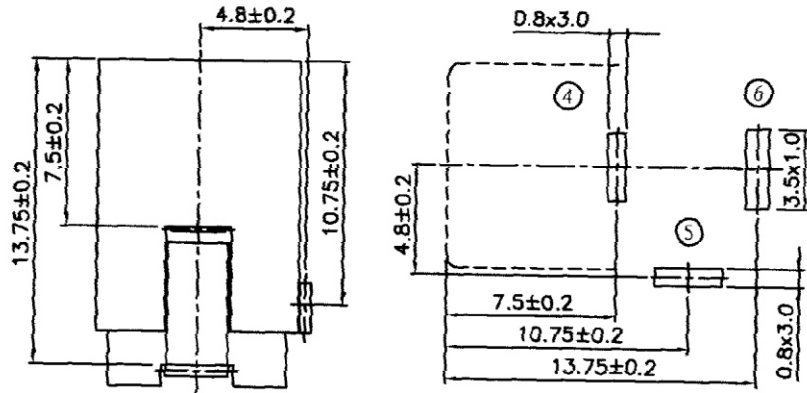
P.C.B. LAYOUT
