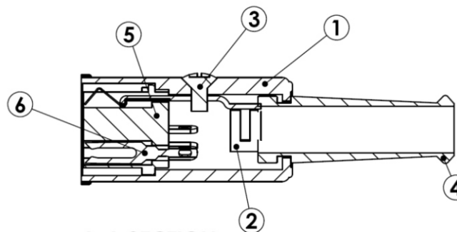
A-A SECTION
