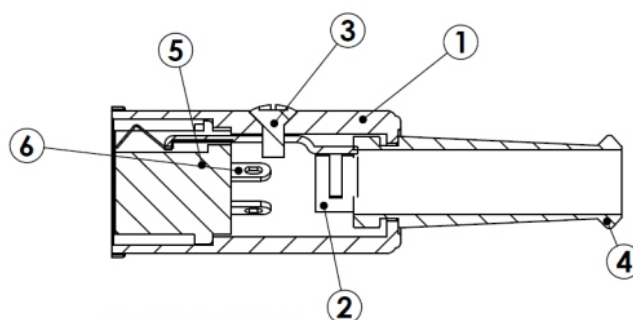
A-A SECTION
