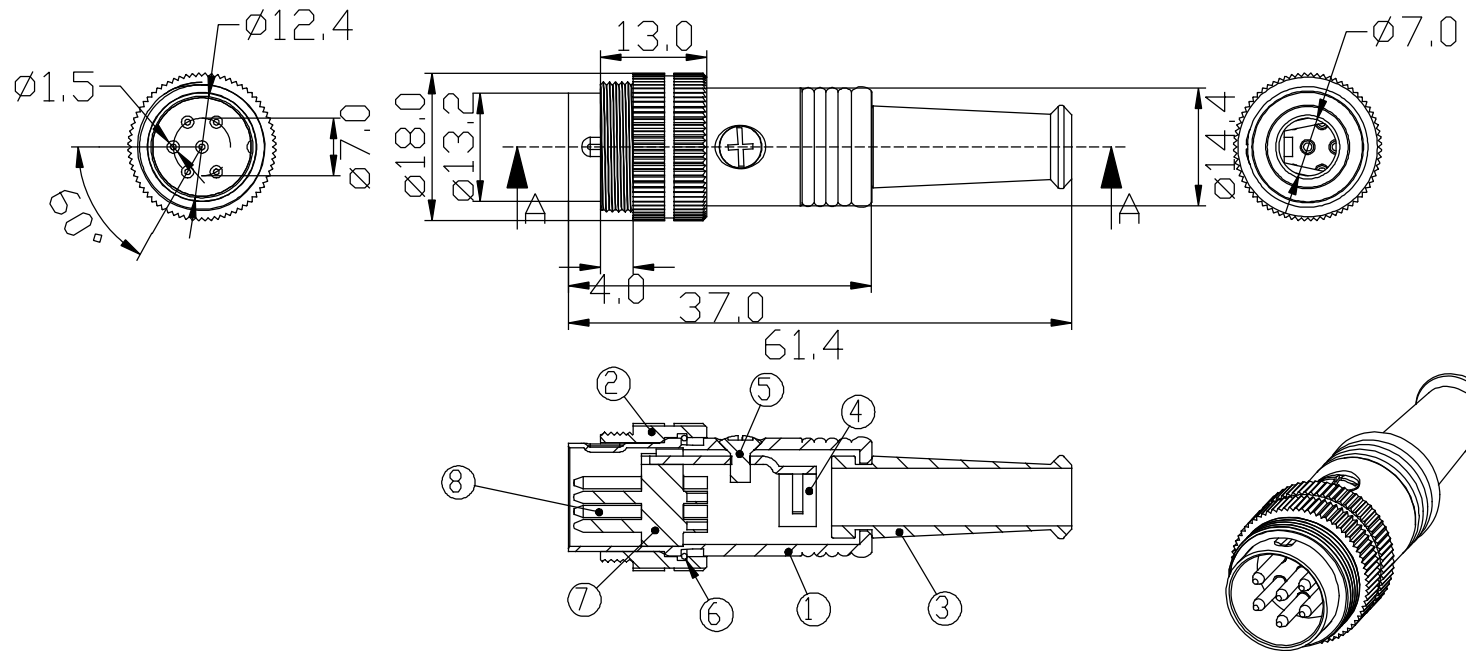
A-A SECTION
