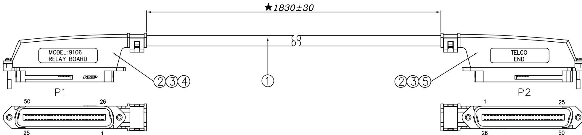
接线图
