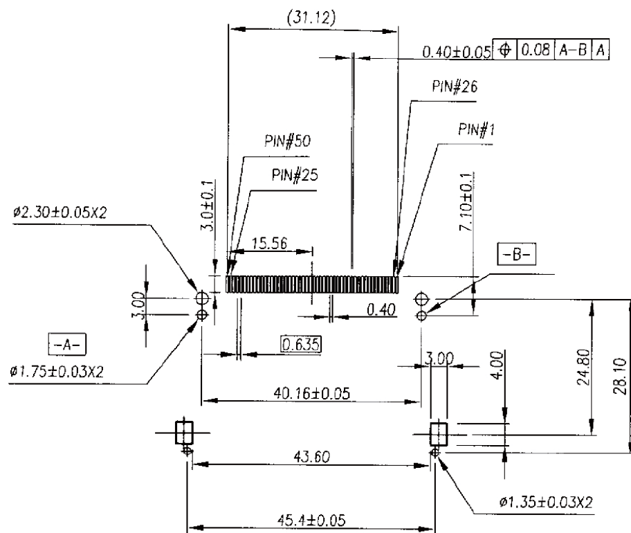
P.C.B Layout
