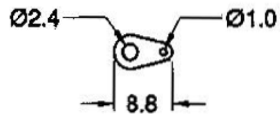
SOLDER LUG
