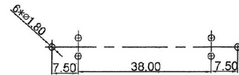
PCB LAYOUT 1:1
