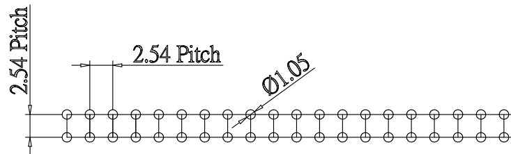
P.C.Board Layout
