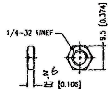
NUT
