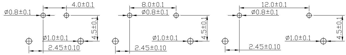
P.C.B LAYOUT
