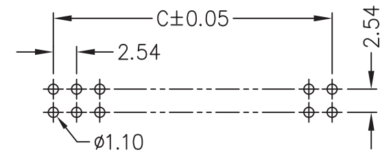
Recommend P.C.B. Layout
