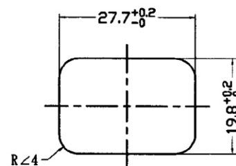
Montageausbruch panel cutout
