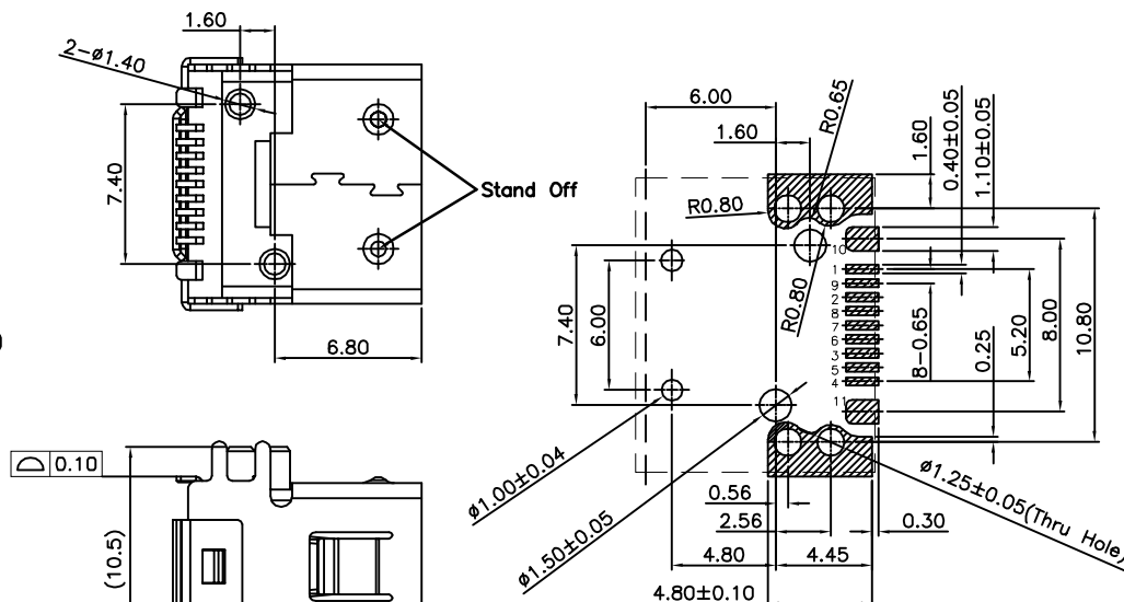
P.C.B Layout
